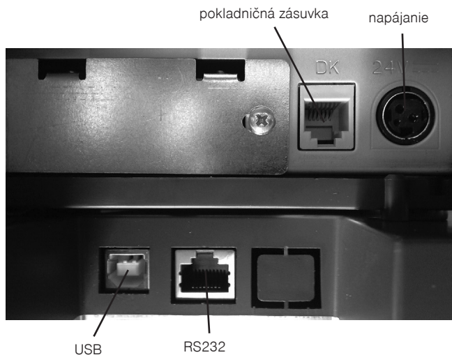
Obrázok 2.5 Komunikačné rozhrania
