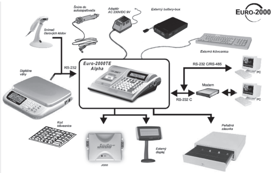
Obrázok 2.3 – Externé zariadenia pripojiteľné k pokladniciam Euro-2000/TE Alpha
