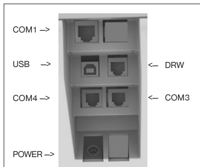
Obrázok 2.2 – Zadné konektory pokladnice Euro-100T
